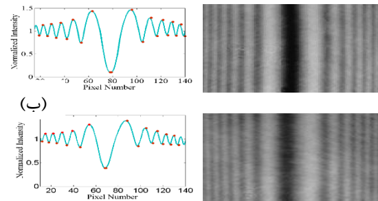
شکل ۵: دو نقش پراش فرنل و نمودار شدت متناظر آن‌ها برای پله ۱۱۰ نانومتری در زوایای الف) ۱۴ درجه و ب) ۵۴ درجه.
