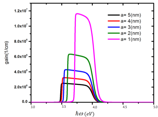
شکل ۸: بهره نوری در چاه کوانتومی نامتقارن دوگانه نیتزیدی به ازای عرض چاه های مختلف.
