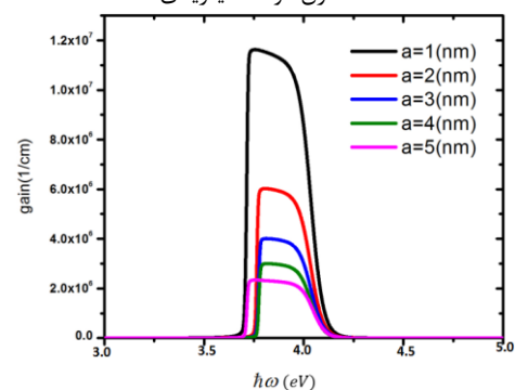
شکل ۱۱: بهره نوری در چاه کوانتومی نامتقارن دوگانه نیتزیدی به ازای عرض سد میانی مختلف.
