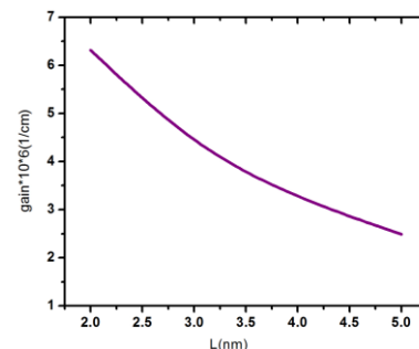
شکل ۱۰: تغییرات بهره نوری با تغییر عرض چاه ها در چاه کوانتومی نامتقارن دوگانه نیتزیدی
