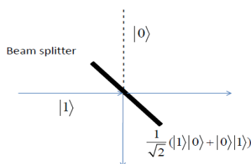
شکل ۱: تولید حالت درهم تنیده از برخورد تک فوتون به شکافنده
