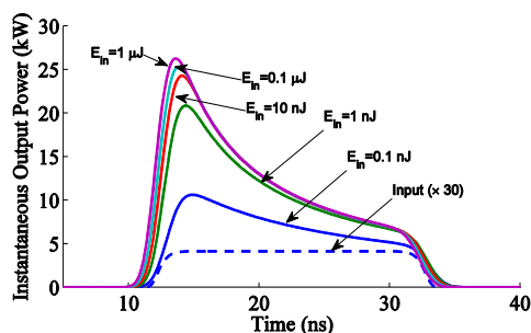
شکل ۳: توان لحظه‌ای خروجی تقویت‌کننده فیبری YDDC برای پالس‌های ورودی سوپر-گوسی با عرض ۲۰ ns و انرژی ۰/۱-nJ تا ۱-μJ.
