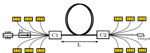
شکل ۱: پیکره بندی یک تقویت کننده فیبری نمونه که از دو طرف پمپ شده. L : طول فیبر YDDC. C1 و C2 : کوپلرهای ورودی و خروجی. LD لیزر دیویدهای پمپ. IS: ایزولاتور ورودی.
