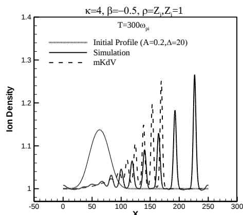
شکل ۲: فرآیند تقسیم پروفایل گوسی به سالیئون‌های یون-صوت غباری در جعبه شبیه‌سازی با n_v = 4801 , n_x = 1024 ، A = 0.2 , \Delta = 20 که dt = 0.01 و گام زمانی L_x = 250
