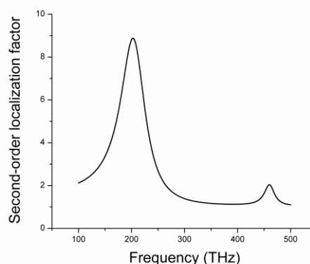
شکل ۱: فاکتور جایگزیدگی مرتبه دوم برای ساختار مورد نظر.
