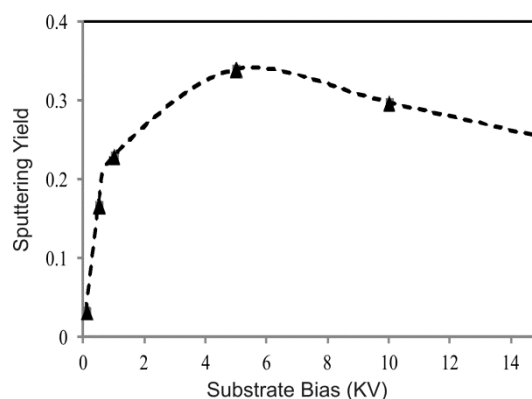
شکل ۲: بازده کندوپاش به ازای ولتاژهای مختلف زیرلایه
