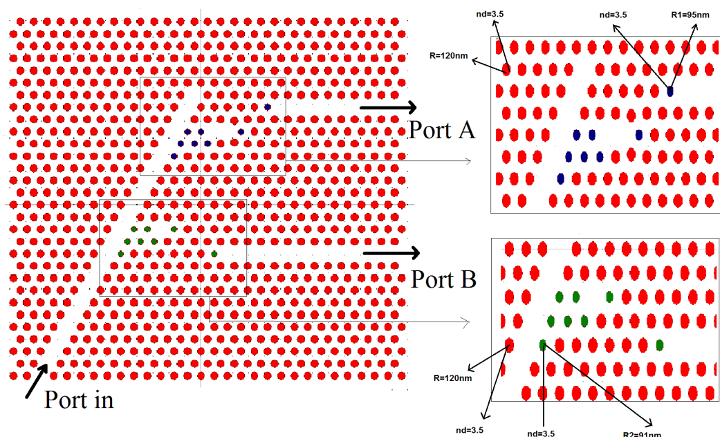
شکل ۲: ساختار افزاره پیشنهادی و بزرگنمایی کاواک‌های آن.
