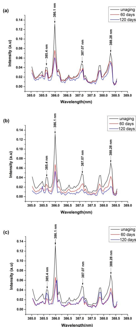
شکل (۳): تغییرات شدت قله‌های بینابی ناشی از کهولت a: ۵۰، b: ۶۰ و c: ۷۰ درجه سانتی گراد
