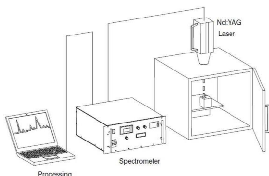
شکل (۱): طرحواره‌ای از چیدمان LIBS
