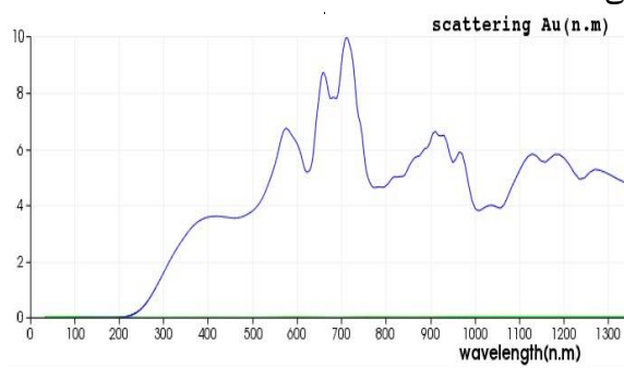
شکل ۲- نمودار پراکندگی هپتامر بدون نانوذرات دی الکتریک کربن
