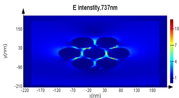
شکل ۴- نمودار شدت میدان الکتریکی هپتامر بدون نانوذرات دی الکتریک در طول موج فانو رزونانس ۷۳۷ نانومتر و اندازه مش ۳ نانومتر
