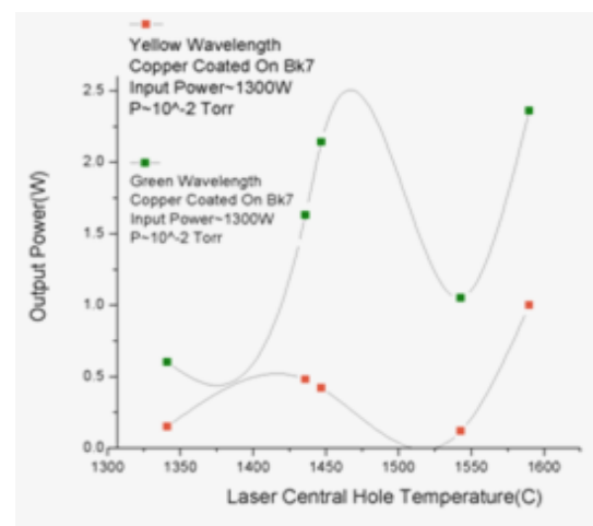
شکل ۵: قرمز: توان خروجی طول موج زرد لیزر بخار مس در حفره مرکزی با آینه مسی و زیر لایه BK7 در فشار 10^{-2} Torr. سبز: توان خروجی طول موج سبز لیزر بخار مس با آینه مسی در حفره مرکزی در فشار 10^{-2} Torr.
