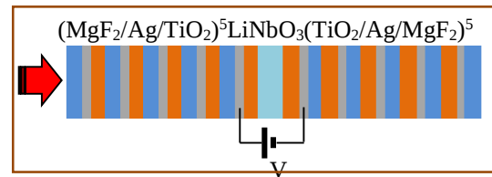
شکل ۱: طرحواره ساختار بلور فوتونی پیشنهاد شده برای طراحی فیلتر نوری کنترل‌پذیر با اعمال ولتاژ خارجی.
