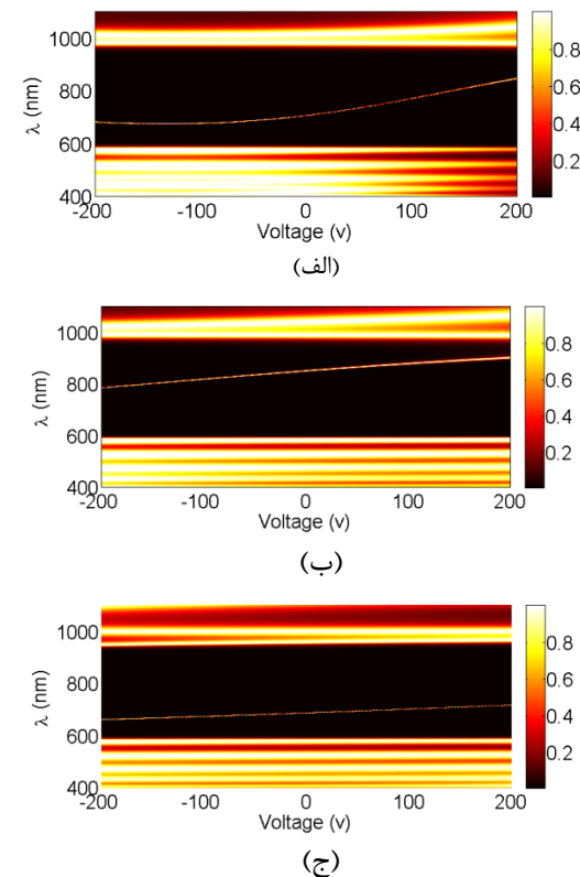
شکل ۳: نمایش رفتار مد نقص در ساختار بلور فوتونی یک بعدی (MgF_2/Ag/TiO_2)^5 LiNbO_3 (TiO_2/Ag/MgF_2)^5 برحسب ولتاژ اعمال شده برای طول موج های مختلف به ازاء سه ضخامت: (الف) ۱۰ نانومتر، (ب) ۶۰ نانومتر و (ج) ۱۶۰ نانومتر لایه نقص.
