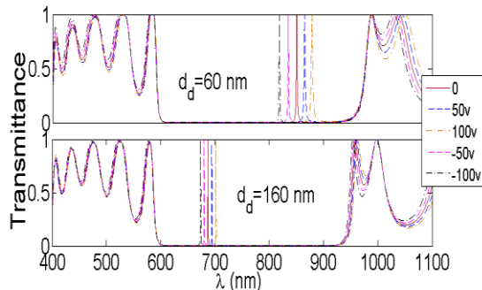
شکل ۲: نمودار تراگسیلندگی برحسب طول موج تابشی از ساختار بلور فوتونی (MgF_2 / Ag / TiO_2)^5 LiNbO_3 (TiO_2 / Ag / MgF_2)^5 جابجایی مد نقص در داخل گاف باند فوتونی با اعمال ولتاژ خارجی قابل مشاهده است.
