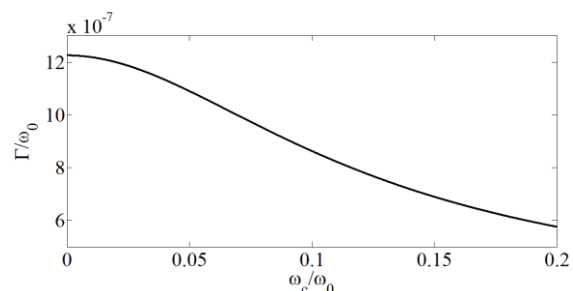
شکل ۱: نحوه تغییرات آهنگ رشد نرمالیزه در پراکندگی بریلوئن رو به جلو نسبت به فرکانس سیکلوترونی نرمالیزه.
