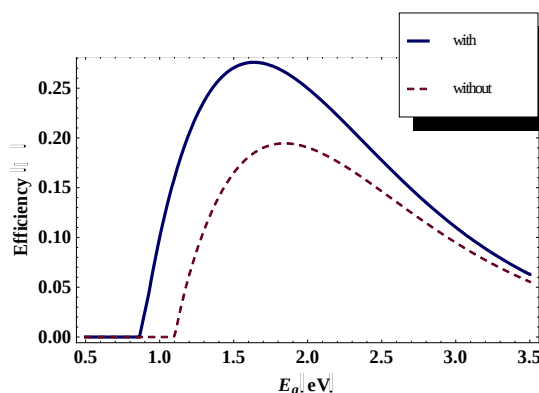
شکل ۳. بازدهی برای سلول دارای بافت سطحی زیر طول موجی و بدون آن.
