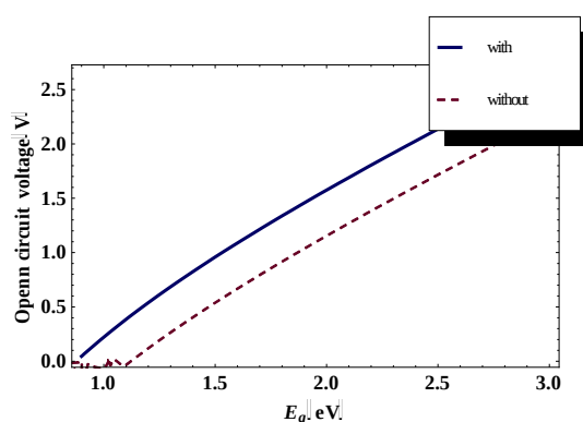
شکل ۲. ولتاژ مدار باز برای سلول دارای بافت سطحی زیر طول موجی و بدون آن.
