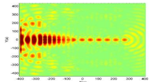
شکل ۳- نمودار توزیع فضایی میدان مربوط به تزویج گر بلور فوتونی مدرج با تغییرات تدریجی ثابت شبکه در دمای ۳۴۲/۸۰۵ کلین
