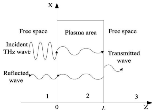
شکل ۱: شماتیک از انتشار موج تراهترتز در لایه پلاسمای محدود شده
