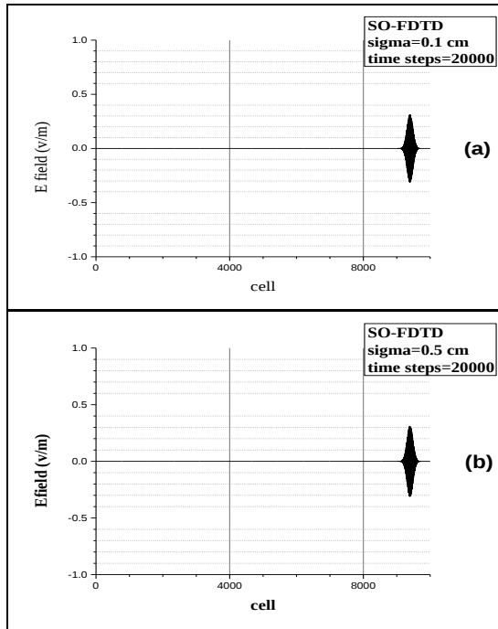
شکل ۵: انتشار موج با فرکانس 1THz در پلاسما، گام زمانی ۲۰۰۰۰ \sigma = 0.5cm (b) . \sigma = 0.1cm (a)
