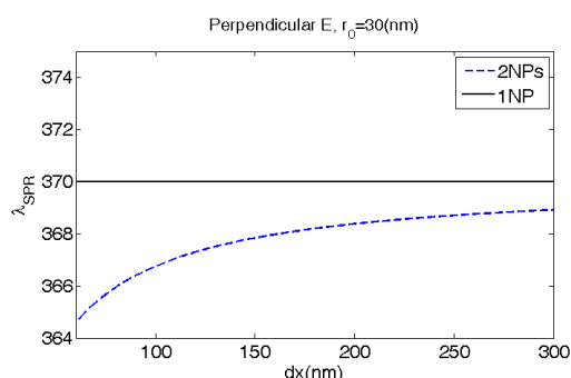
شکل ۷ طول موج تشدید پلاسمون سطحی برای دو نانوذره نقره به شعاع 30\text{nm} برحسب فاصله ذرات.
