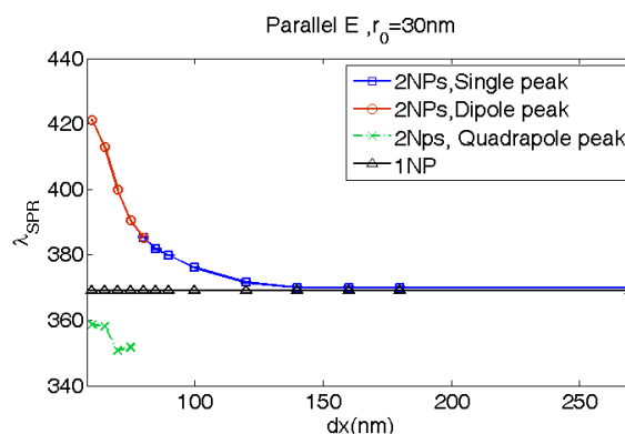
شکل ۶ طول موج تشدید پلاسمون سطحی برای دو نانوذره نقره به شعاع 30\text{nm} برحسب فاصله ذرات.
