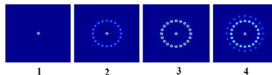
شکل ۲: نحوه‌ی انتشار نور در آرایه در حالت منظم زمانی که ورودی در فیبر مرکزی اعمال شده است.
