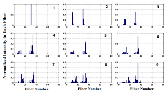
شکل ۹: نمایی از نحوه‌ی انتشار نور در آرایه برای بی‌نظمی S=0.6 برای حالتی که ورودی به یک فیبر از حلقه‌ها اعمال شده است.
