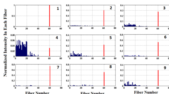
شکل ۶: نمایی از نحوه‌ی انتشار نور در آرایه برای بی‌نظمی S=0.6 برای حالتی که ورودی به فیبر مرکزی اعمال شده است
