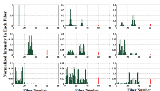
شکل ۷: نحوه‌ی انتشار نور در آرایه برای حالت منظم، برای حالتی که ورودی به یک فیبر از حلقه‌ها اعمال شده است.
