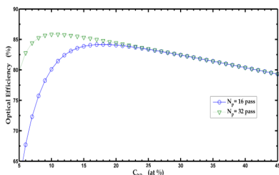
شکل ۷: نمودار بازده اپتیکی بر حسب غلظت ماده فعال برای تعداد عبور ۱۶ و ۳۲ بار
