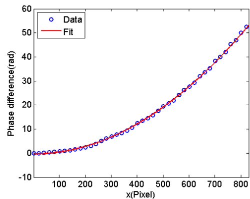
شکل ۴: نمایه توزیع اختلاف فاز دو موج تداخلی در امتداد شعاع. دایره‌های آبی و خط توپر قرمز به ترتیب نتایج تجربی و منحنی درجه دو برازش شده بر آن را نشان می‌دهند.
