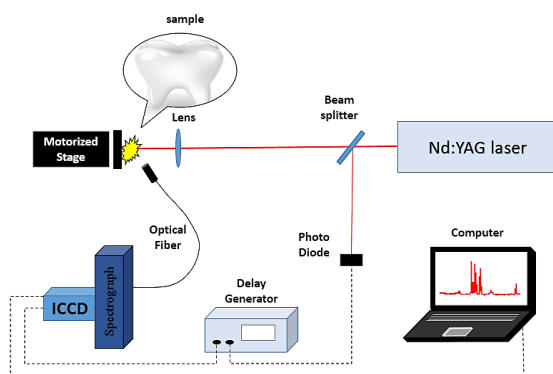
شکل ۱: چیدمان آزمایش
