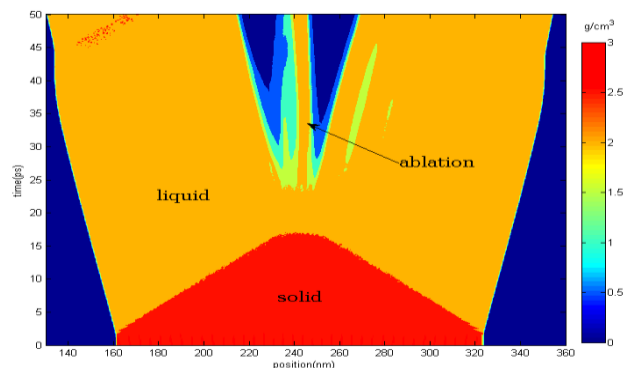
شکل ۷: تغییرات فاز در قطعه برای 2,00 \text{ J/m}^2 ، زمان بر حسب مکان
