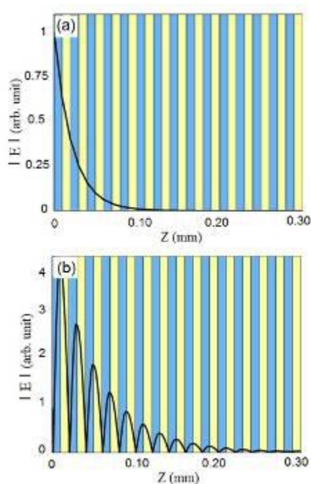
شکل ۵: توزیع میدان الکتریکی امواج الکترومغناطیسی در درون بلور فوتونی و برای دو فرکانس (a) f = 0.67 THz و (b) f = 4/2 THz برای تابش عمودی، T = 300 K و \mu_c = 0.2 eV.
