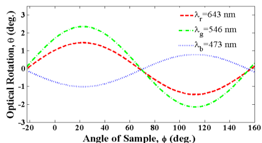
شکل ۳: چرخش نوری بر حسب زاویه چرخش نمونه‌ی ایجاد شده با پرتو قطبیده‌ی 22/5^\circ راستگرد (R) و چپگرد (L) برای سه طول موج مختلف.
