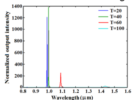
شکل ۴: نمودار بهنجار خروجی فیلتر برای دماهای مختلف از ۲۰ تا ۱۰۰ درجه سانتی-گراد.
