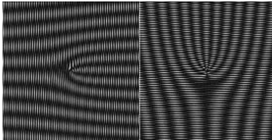
شکل ۳: نقش ماره‌ی ناشی از برهم‌نهی دو توری چنگالی با دوران زوایای نسبی راست: \alpha < 1 و چپ: \alpha - \pi < 1 . توری‌ها دارای تعداد انشعاب l_1 = 5 و l_2 = 2 هستند.
