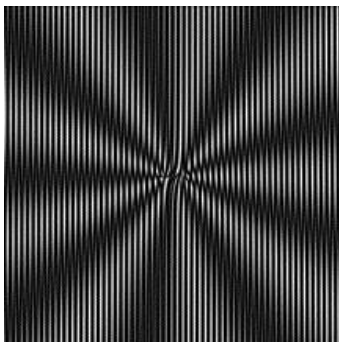
شکل ۲: نقش ماره‌ی ناشی از برهم‌نهی دو توری چنگالی با گام برابر که راستای کلی خطوط آن‌ها با هم موازی است و l_1 = 5 و l_2 = -4 . تعداد پره‌ها یا فریزهای ماره در این نقش ۹ است.
