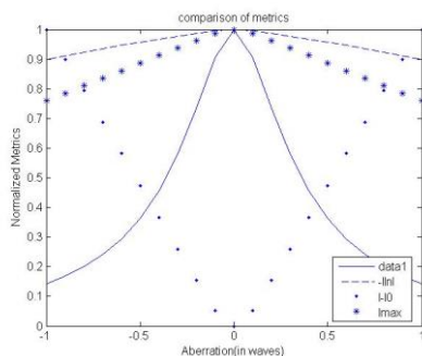
شکل ۱: مقایسه‌ی متریک‌های I \ln I , I - I_0 , I_{max} و نسبت اشترل با تغییر دامنه‌ی ابیراهی کروی
