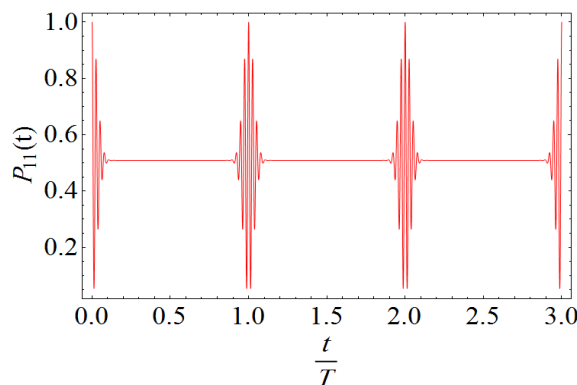
شکل ۱: احتمال P_{11}(t) برحسب \frac{t}{T} برای توزیع فوتونی متناظر با حالت همدوس استاندارد و به ازای مقادیر \frac{\omega_a}{\nu}=2 و N=25 .
