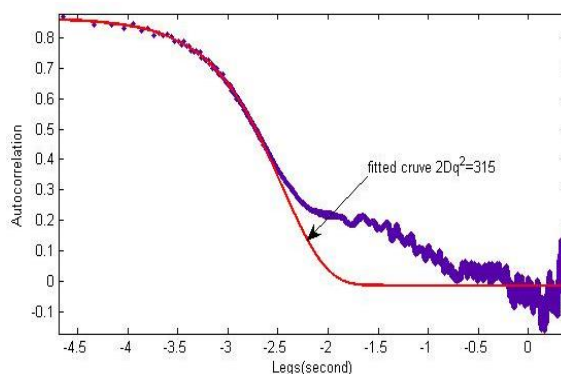
شکل ۲: تابع خودهمبستگی شدت برای ذرات پلی‌استایرن با قطر اسمی 1\mu\text{m} و نمودار برازش شده بر آن.
