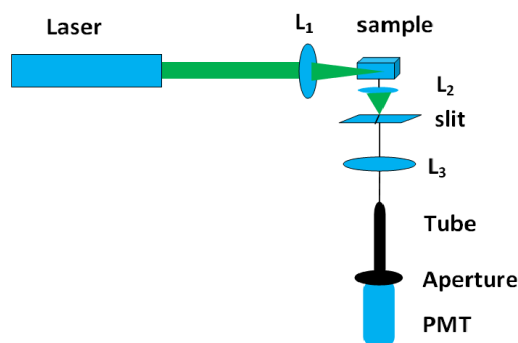
شکل ۱: چیدمان آزمایش پراکندگی دینامیکی نور برای اندازه‌گیری توزیع اندازه‌ی ذرات
