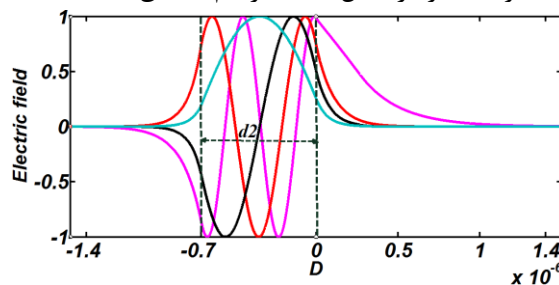
شکل ۶: توزیع میدان الکتریکی در موجبر ۵ لایه معکوس برای مدهای مختلف.
