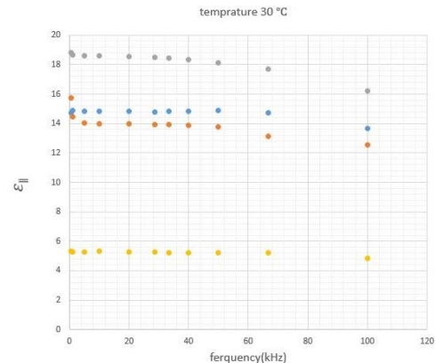
شکل ۳: وابستگی مولفه موازی ثابت دی الکتریک به فرکانس و غلظت نانو ذرات سیلیکا
