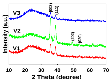
شکل ۲: طیف XRD لایه های اکسید مس با حجم های مختلف محلول.
