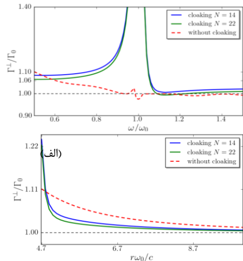
شکل ۴: نمودار بخش عمودی گسیل خودبخودی (۱۲) بر حسب (الف) فرکانس بدون بعد \omega_A / \omega_0 و (ب) فاصله بدون بعد r\omega_0 / c . ترسیم شده است. در اینجا \gamma / \omega_0 = 0.0 ، \omega_p / \omega_0 = 0.1 و a_{N-1}\omega_0 / c = 3 ، a_1\omega_0 / c = 4.5 و r_A\omega_0 / c = 4.7 است.
