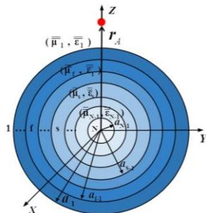
شکل ۱: نمایی از پوشش ماتموادی ناپدیدکننده.
