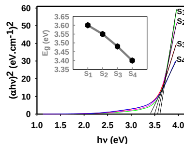
شکل ۴: تغییرات (\alpha h\nu)^2 بر حسب انرژی فوتون‌ها.
