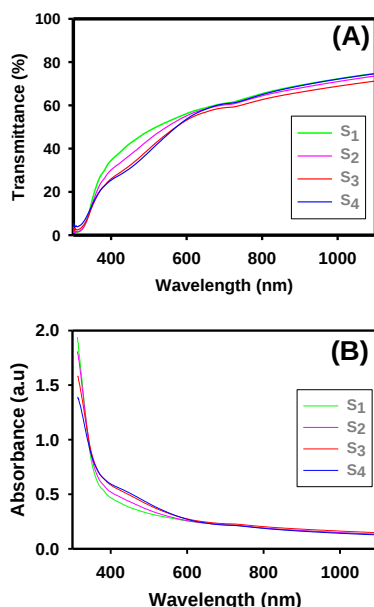
شکل ۳: (A) طيف عبور و (B) طيف جذب اپتيکي نمونه‌هاي مورد بررسي.
