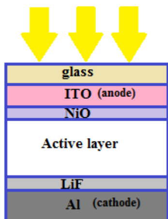
شکل ۱: ساختار سلول خورشیدی آلی متشکل از لایه فعال P3HT:PCBM و PCPDTBT:PCBM
