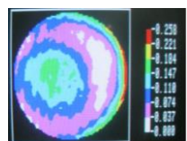
شکل ۱۷: ناهمواری جبهه‌موج حاصل از آزمون MTF بر روی سامانه‌ی تصویربرداری پس از انجام تنظیمات
