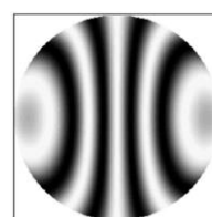
شکل ۹: الگوی تداخلی بیانگر افت کیفیت در سامانه، در نتیجه‌ی ایجاد عدم هم‌راستائی به میزان TLB=0.1^\circ در لنز اول
