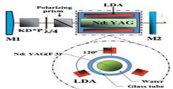
شکل ۱: چیدمان لیزر کلید زنی Q
