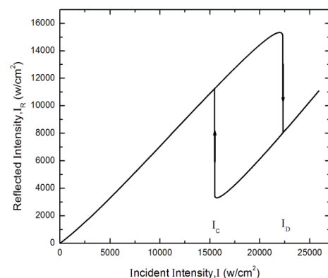
شکل (۸): نمودار شدت بازتابی بر حسب شدت ورودی با
