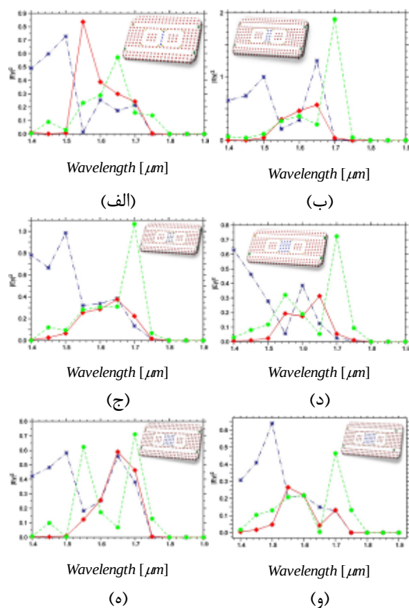
شکل ۴: پاسخ طیفی توان انتقالی ساختار تشدیدگر حلقوی دوتایی بر بلور فوتونی در هندسه موازی، نمودار خطی (کانال C)، خط تیره (کانال D) و خط تیره - دو نقطه (کانال B)
