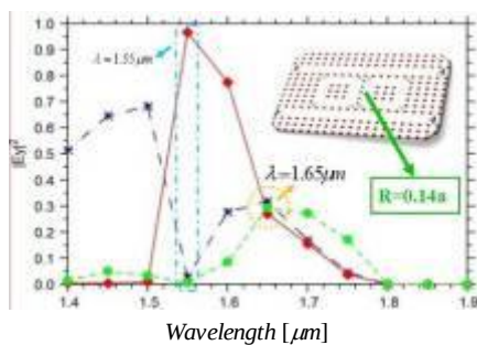
شکل ۵: بررسی تاثیر تغییر شعاع میله‌های توزیع گر بر روی پاسخ طیفی توان انتقالی تشدیدگر حلقوی دوتایی بلور فوتونی در هندسه موازی
