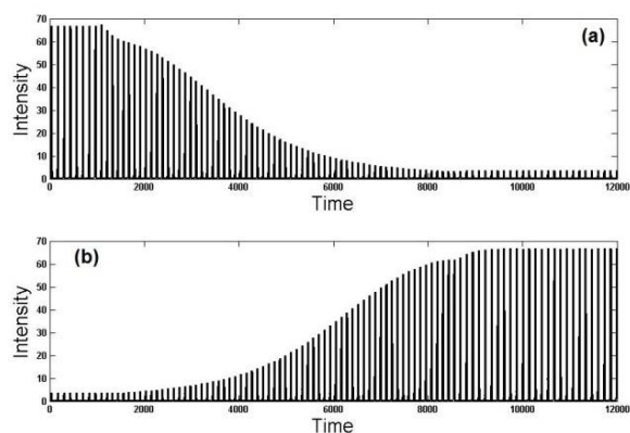
شکل ۳: تحول زمانی شدت میدان الکتریکی در طی فرایند حرکت کنترل شده سولیتون کاواک تپنده، در (a) مکان اولیه سولیتون کاواک (10,0) و (b) مکان نهایی سولیتون کاواک تپنده (0,-10) نشان داده شده است.
