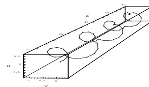
Figure ۲ نمودار ۳ بعدی مسیر حرکت الکترون از میان ویگنر ویسلر پلاسمایی
