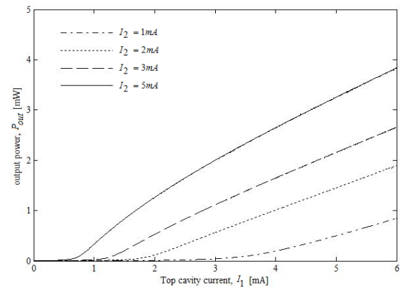
شکل ۴: منحنی توان نوری بر حسب جریان تزریق در کاواک بالا
