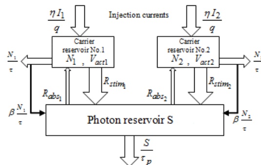
شکل ۲: نمایش مفهومی معادلات نرخ شامل روابط (۱) الی (۳)
