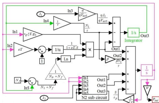
شکل ۳: ساختار مدل طراحی شده حاکم بر رفتار لیزر CRVCL
