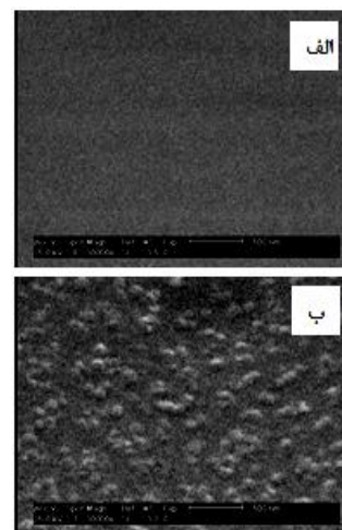
شکل ۳: تصویر SEM پلیمر PADC تابش‌دهی شده با لیزر ArF با شاریدگی 50 \text{ mJ/cm}^2 (الف) و 3000 \text{ mJ/cm}^2 (ب) تب.
