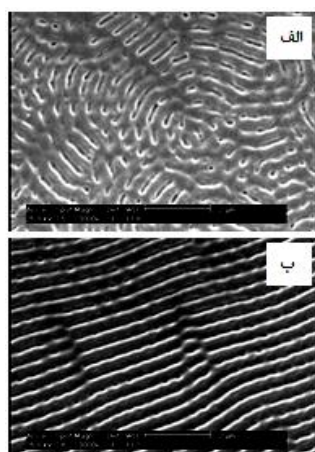
شکل ۴: تصویر SEM برای پلیمر PADC تابش‌دهی شده با لیزر ArF با شاریدگی 50 \text{ mJ/cm}^2 (الف) و 1000 \text{ mJ/cm}^2 (ب) تب.
