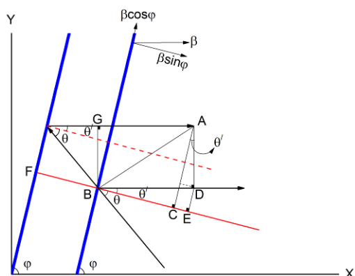
شکل ۱: ساختار هندسی برای محاسبه طول پالس پس از بازتاب.
