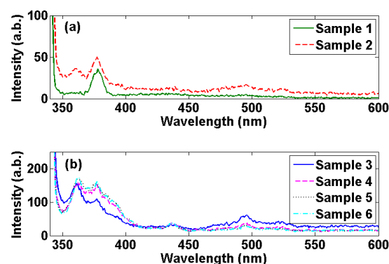
شکل ۴: طیف فلومینسانس نانوذرات اکسید روی تولید شده در (a) طول موج ۵۳۲ نانومتر (b) طول موج ۱۰۴۶ نانومتر.
