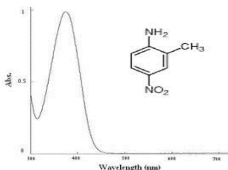
شکل ۱: طیف جذب رنگینه DR1
