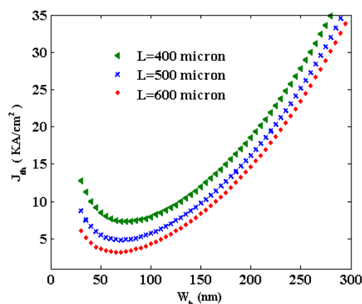
شکل ۳: منحنی تغییرات چگالی جریان آستانه بر حسب W_b
