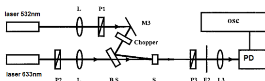
شکل ۱: چیدمان دوشکستی القایی: P 2 : پلاریزور، L 3 : لنز، M 3 : آینه، S: نمونه، F: فیلترسبز، PD: آشکارساز، OSC: اسیلوسکوپ، B.S: شکافنده پرتو.
