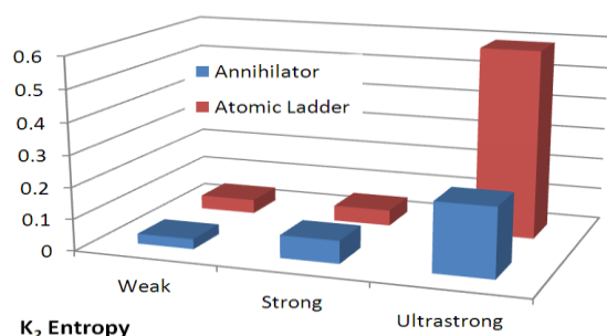
شکل ۴: محاسبه‌ی آنتروپی کولموگوروف در رژیم‌های تزویج متفاوت.
