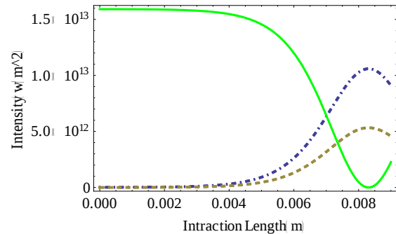
شکل ۴: شدت سیگنال (خط نقطه)، پمپ (خط) و ایدلر (خط چین) بر حسب طول کریستال
